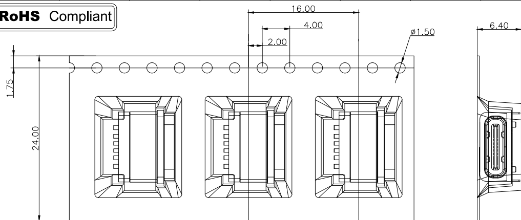
① 产品入载带示意图
