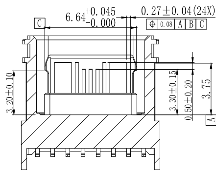
截面B-B
