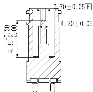
截面A-A
