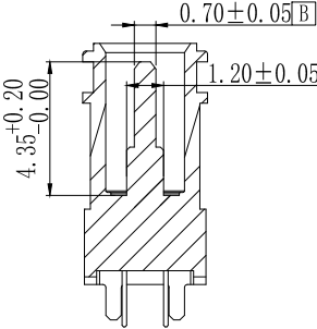
截面A-A
