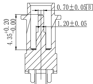
截面A-A
