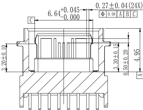
截面B-B
